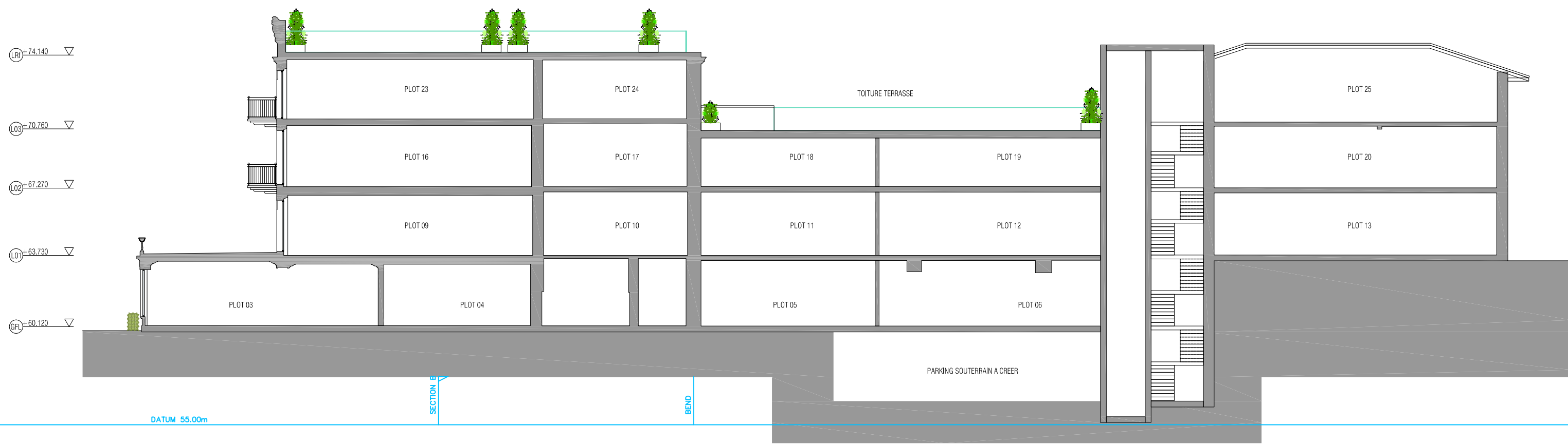
- COUPE B-B - 1:200 -
